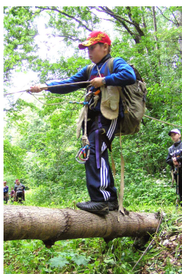
навесная переправа
